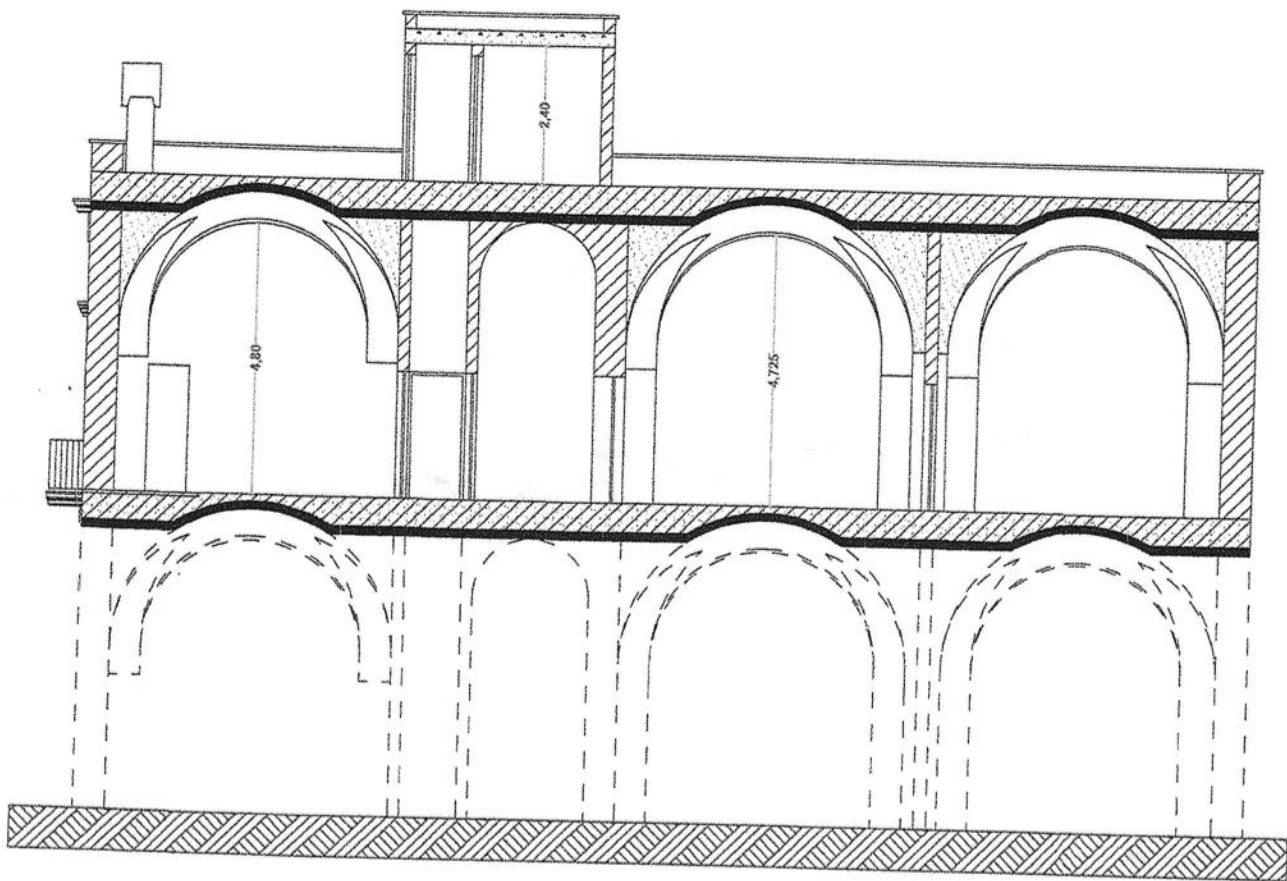
SEZIONE A-A STATO DI FATTO
